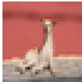
DPP (ours)
